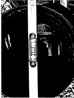
Photos : Vérification de la collecte des effluents et mesure de l'horizontalité sur un regard de visite
